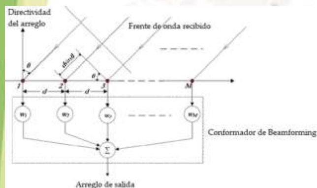
Figura 4. Arreglo lineal uniforme. Ángulo de arribó al transmisor para la selección del peso específico [18].
