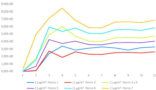
Fig. 8 Ladrillera 2. Concentraciones de PM 10 de cada horno a los receptores.
