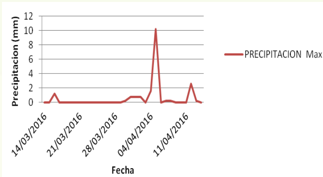
Fig. 6 Información meteorológica procesada variable "precipitación máxima" para ladrillera 2.
