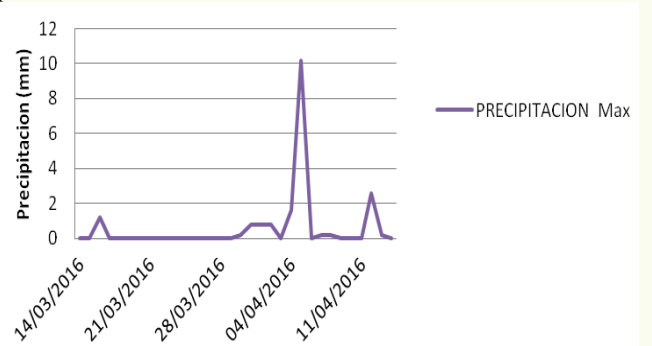
Fig. 3 Información meteorológica procesada variable "precipitación máxima" para ladrillera 1.
