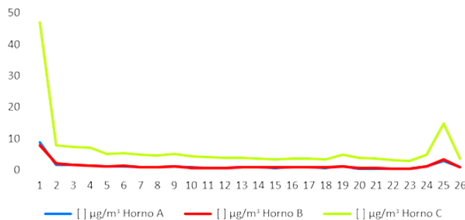
Fig. 7 Ladrillera 1. Concentraciones de PM 10 de cada horno a los receptores.
