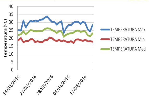
Fig. 1 Información meteorológica procesada variable temperatura para ladrillera 1.
