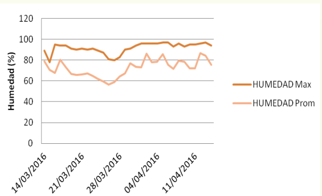
Fig. 2 Humedad información meteorológica procesada variable humedad para ladrillera 1.
