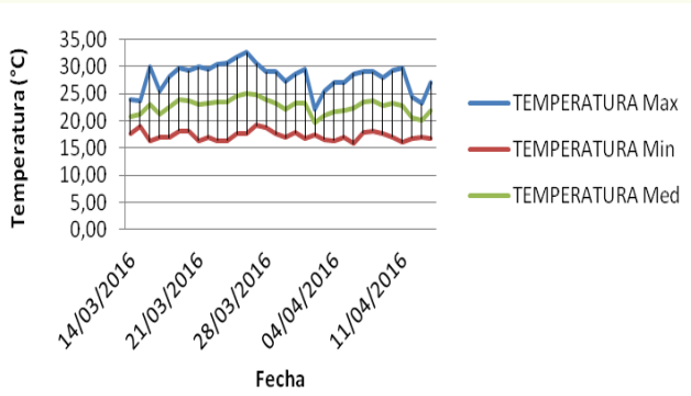
Fig. 4 Información meteorológica procesada variable temperatura para ladrillera 2.
