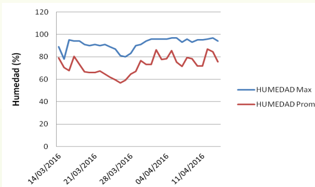
Fig. 5 Humedad información meteorológica procesada variable humedad para ladrillera 2.
